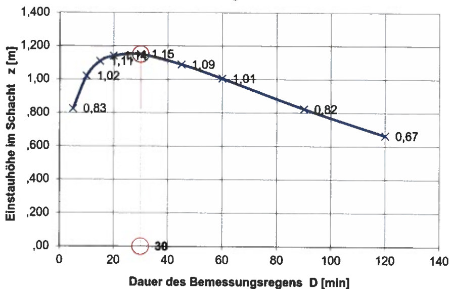
Versickerungsschacht
