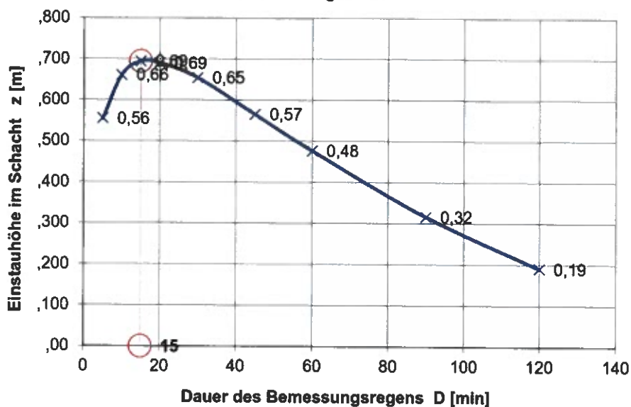
Versickerungsschacht
